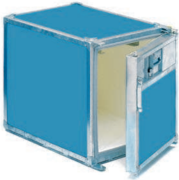
Contenedor Isotérmico apilable 170 lts. con soporte placa eutéctica. Med, 800x600.680 mm. Azul
