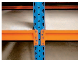
Detalle de Puntal y Larguero " Z " con soporte de tablero de Aglomerado.
